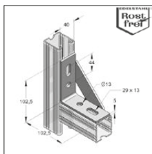
Łącznik kątowy 40/5 z czterema otworami
