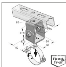
Łącznik przegubowy
