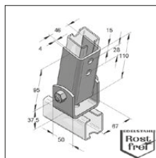
Uchwyt przegubowy
